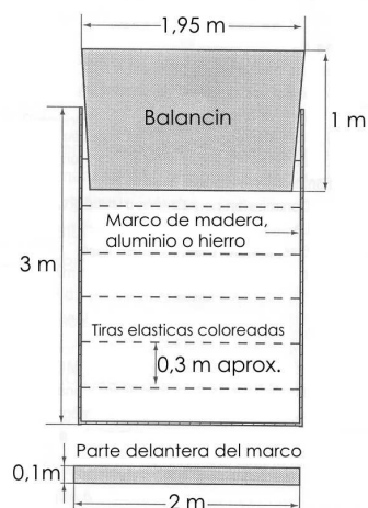
DETALLE DEL MARCO PARA EL SALTO DE LONGITUD
